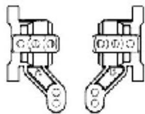
Rear upright A/B 六角軸止 A/B
